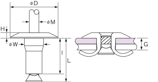
(Large flange)
