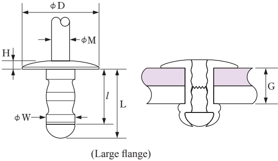
(Large flange)
